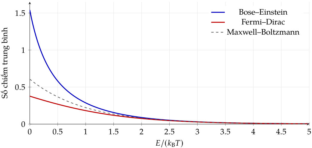
Hình 1: So sánh ba phân bố tại cùng nhiệt độ và -\mu/(k_{\text{B}}T) = 0.5 . Phân bố Bose–Einstein tăng mạnh ở vùng năng lượng thấp, trong khi nguyên lý Pauli giữ số chiếm Fermi–Dirac dưới một. Ở năng lượng cao, cả hai tiến gần giới hạn Maxwell–Boltzmann.
