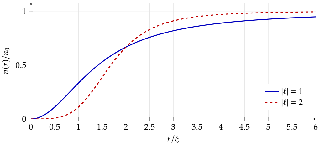
Hình 10: Các hồ sơ gần đúng minh họa sự suy giảm mật độ tại lõi vortex. Vortex có số quẩn lớn có lõi rộng hơn và chi phí động năng lớn hơn.
